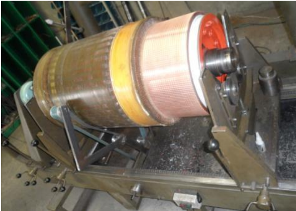
Balanceamento dinâmico
